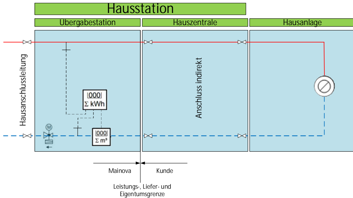
Abbildung 5-1: Skizze Hausstation
